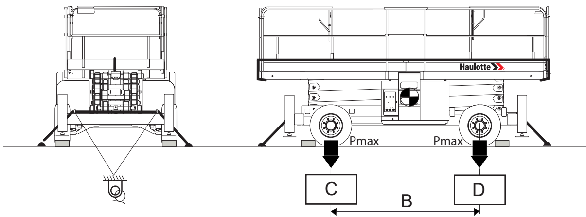
Погрузочные характеристики
