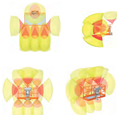
Рис. 32. Зоны покрытия уровня 2 SkySense (3 штанги)
