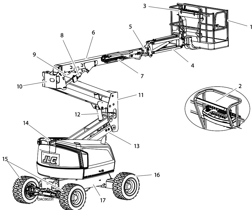
Рис. 1. Основные элементы конструкции
