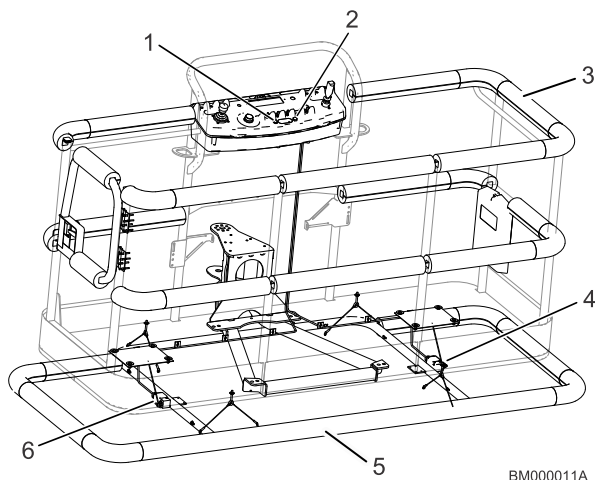
Рис. 36. Система Soft Touch
