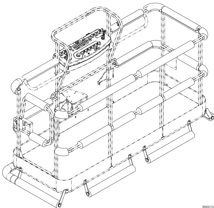
Рис. 34. Амортизирующая обивка бампера платформы
