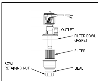
Рис. 37. Узел фиксатора фильтра Kubota
