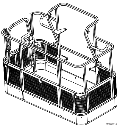
Рис. 26. Сетка платформы для крепления на среднем поручне
