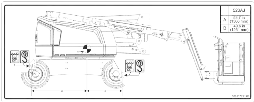
Рис. 12. Схема подъема 520AJ
