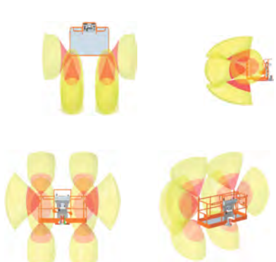
Рис. 28. Зоны покрытия уровня 1 SkySense (2 штанги)
