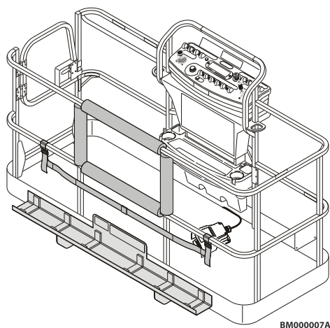
Рис. 26. Система SkyGlazier
