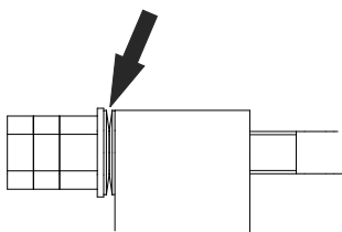
Рис. 14. Неправильный зазор
