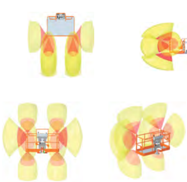
Рис. 19. Зоны покрытия уровня 1 SkySense (2 штанги)
