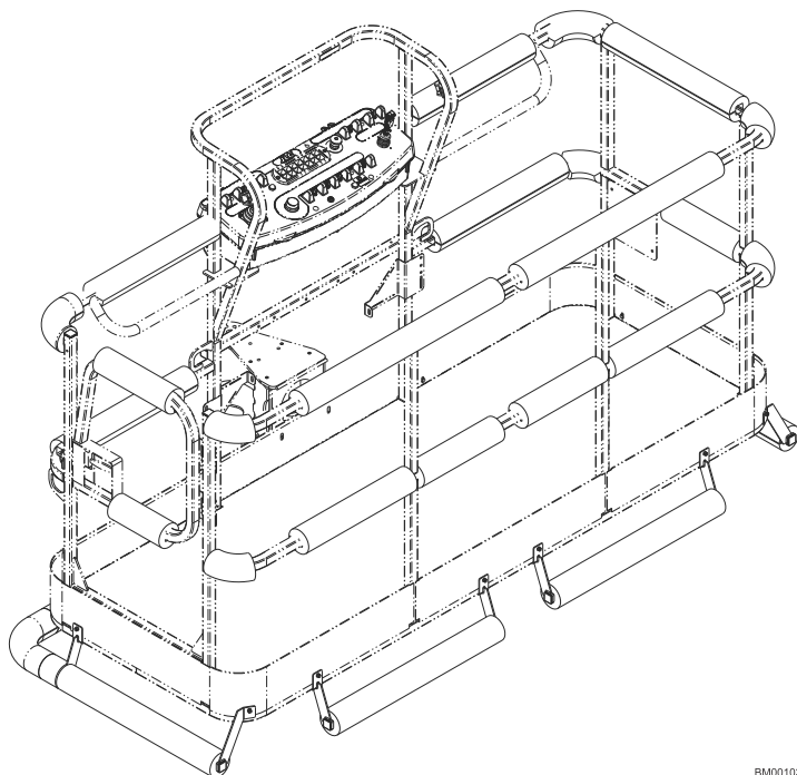
Рис. 21. Амортизирующая обивка бампера платформы
