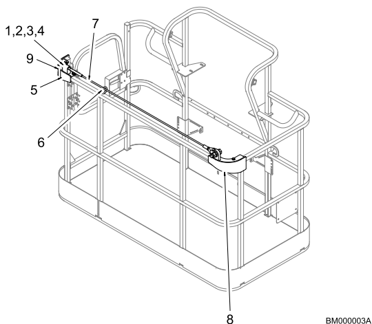
Рис. 13. Внешняя страховочная система с болтовым креплением
