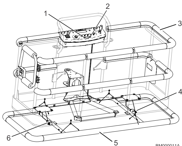
Рис. 22. Система Soft Touch
