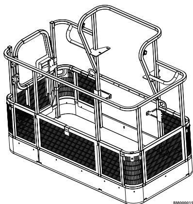
Рис. 21. Сетка платформы для крепления на среднем поручне
