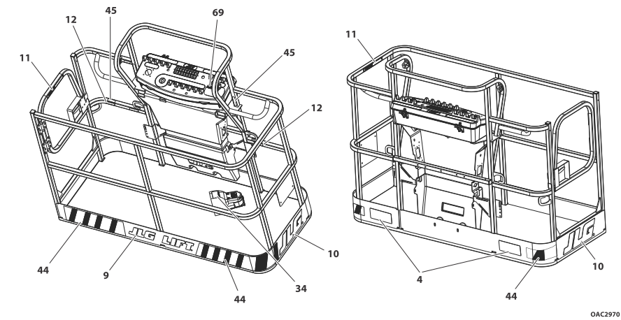
Рис. 13. Расположение наклеек — вид 4
