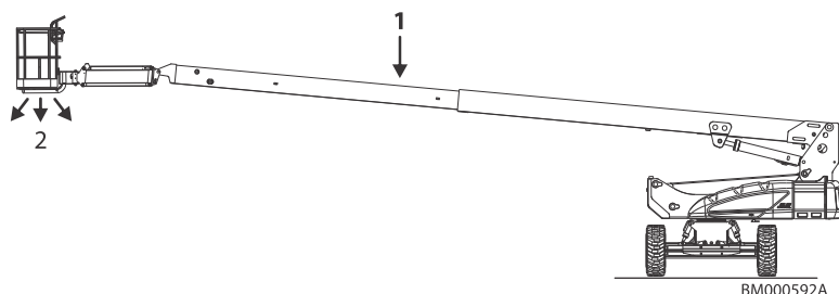
Рис. 6. Положение минимальной устойчивости к опрокидыванию вперед
