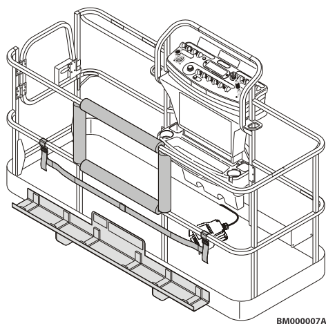
Рис. 27. Система SkyGlazier
