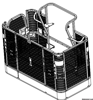
Рис. 22. Сетка платформы для крепления на верхнем поручне
