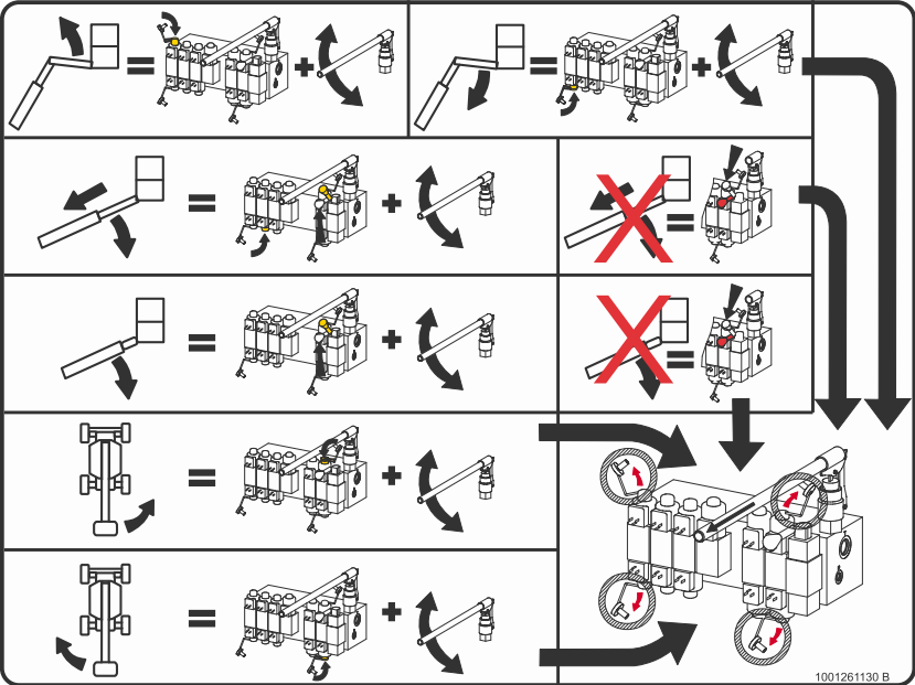
Рис. 15. Табличка клапана ручного опускания
