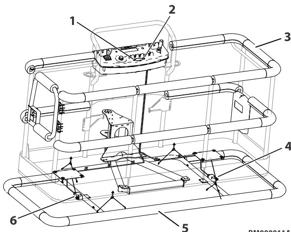
Рис. 28. Система Soft Touch
