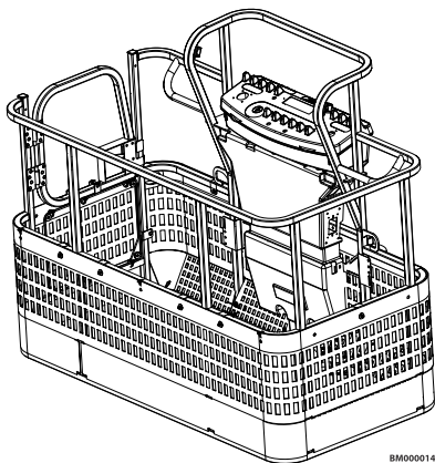
Рис. 18. Тканевая сетка для крепления на среднем поручне
