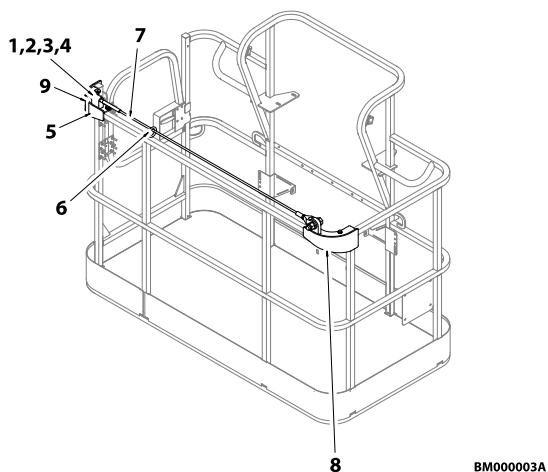
Рис. 17. Внешняя страховочная система с болтовым креплением
