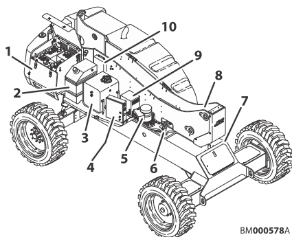
Рис. 1. Основные обозначения — лист 1 из 3
