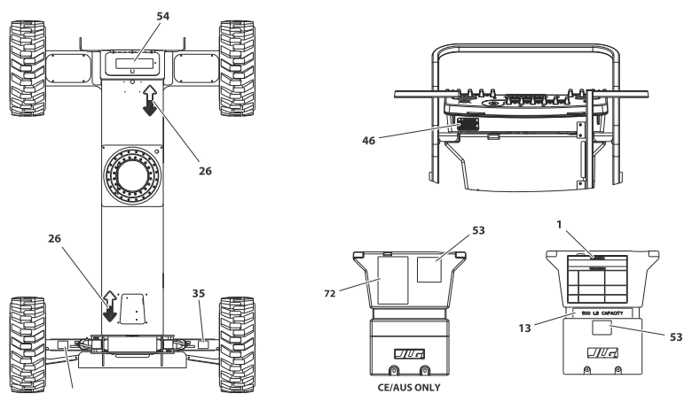
Рис. 14. Расположение наклеек — вид 5
