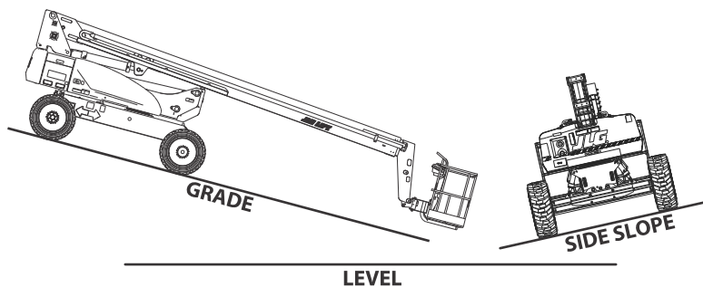
Рис. 9. Уклон/поперечный уклон
