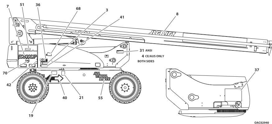
Рис. 10. Расположение наклеек — вид 1
