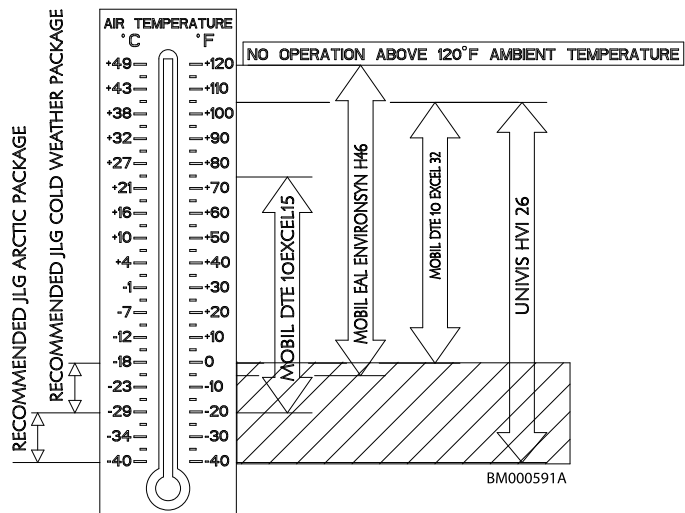
Рис. 29. Спецификации рабочей температуры гидравлической системы
