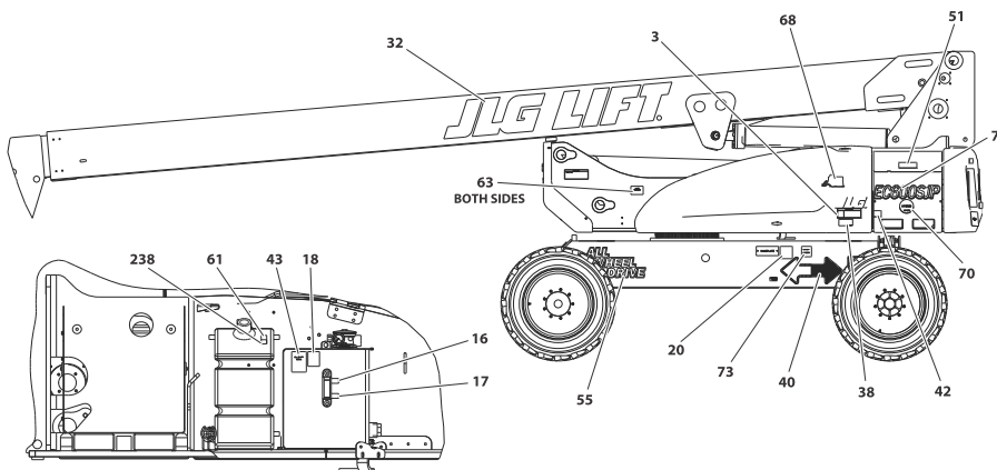
Рис. 11. Расположение наклеек — вид 2
