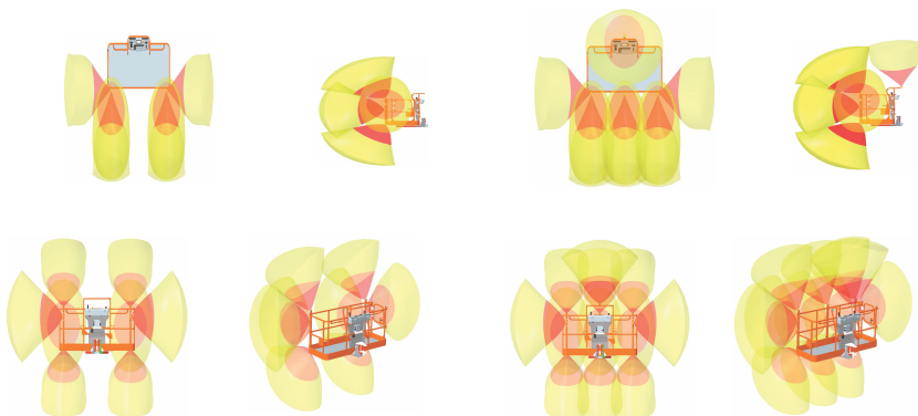
Рис. 25. Зоны покрытия уровня 1 SkySense (2 штанги)
