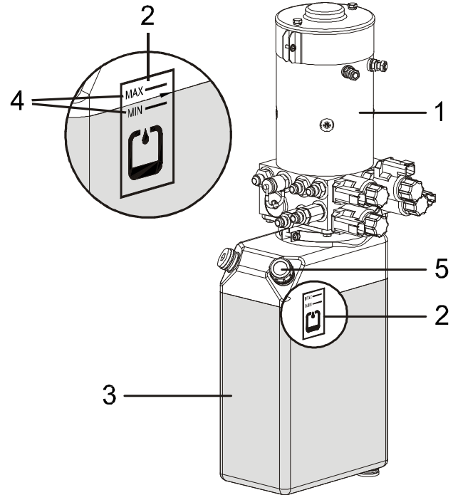
Рис. 5-8. Проверка гидравлического масла - 10E/26E
