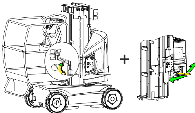
Рис. 3-8. Клапан ручного подъема стрелы и мачты — 20E
