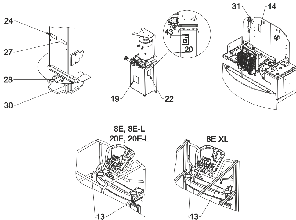
Рис. 5-12. Местоположение наклеек - 8E/20E, все рынки — лист 3/3
