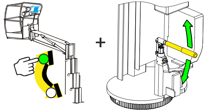
Рис. 3-13. Клапан ручного подъема стрелы и мачты — 26E
