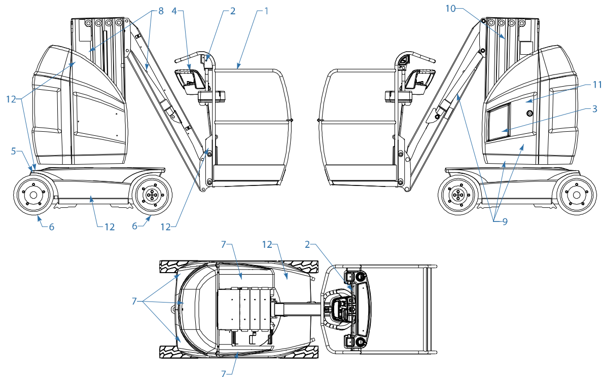
Рис. 2-2. Ежедневный общий осмотр - 10E/26E
