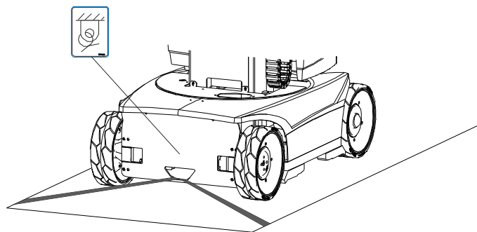
Рис. 3-20. Крепление машины - 8E/20E
