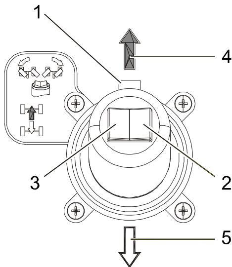
Рис. 3-18. Ручки рулевого управления/движения
