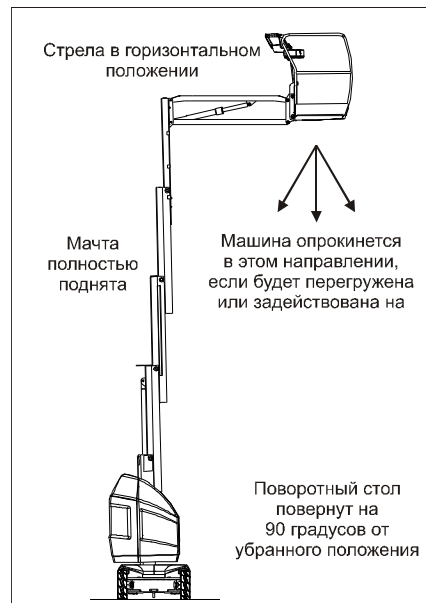
Рис. 3-2. Положение наименьшей передней устойчивости
