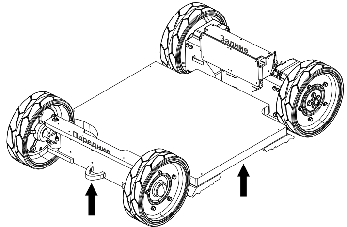
Рис. 5-26. Точки для поддомкрачивания
