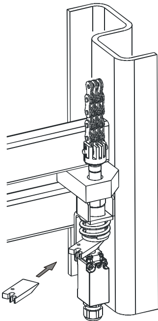
Рис. 5-27. Датчики провисания/поломки
